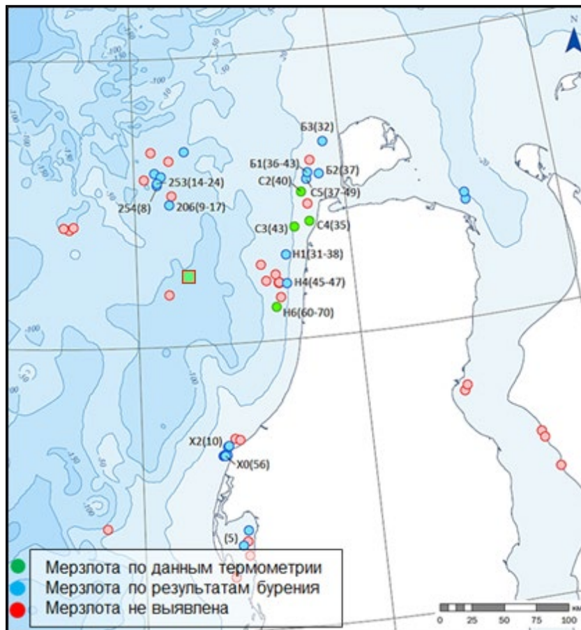
Рисунок 3.3-3 Карта фактического материала результатов вскрытия мерзлых грунтов по результатам инженерно-геологического бурения на Ямальском шельфе Карского моря (зелёным квадратом с красной обводкой выделен участок работ)
