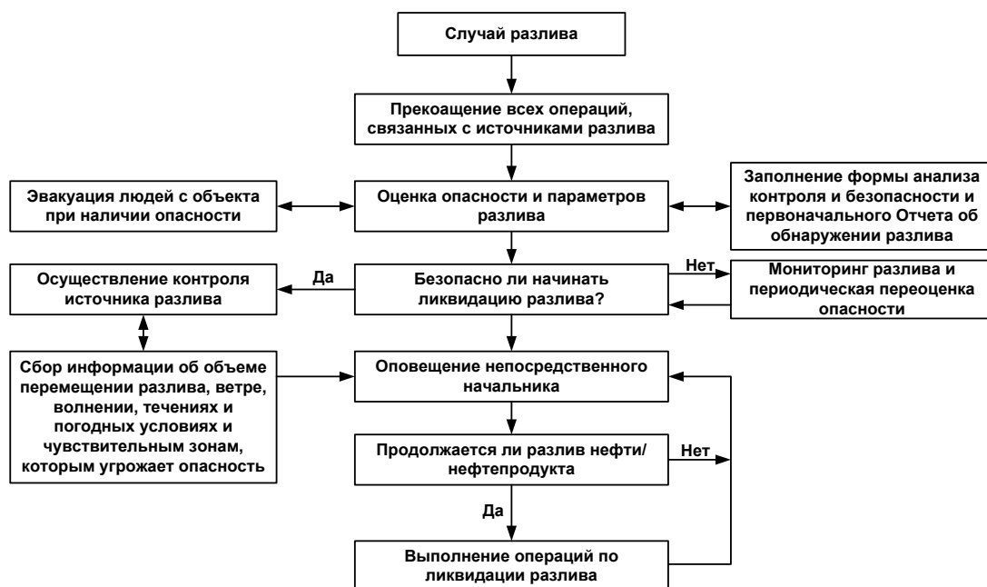
Рисунок 5.9-1 Схема ликвидации разлива нефтепродукта
