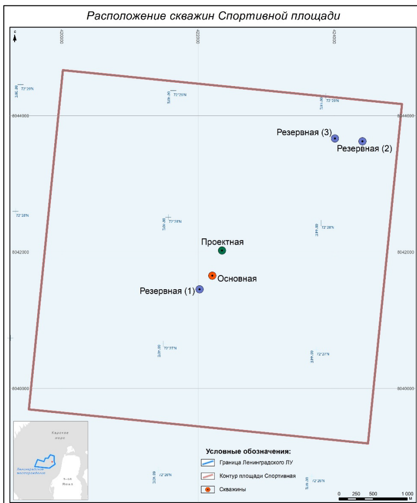
Рисунок 3.3-6 Расположение скважин в пределах Спортивной площадки
