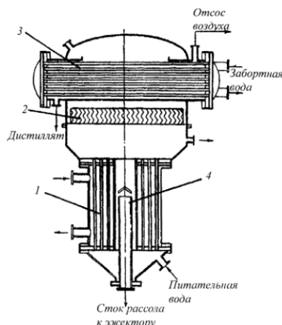
Рисунок 4.4-3 Конструктивная схема опреснителя типа «Д»
